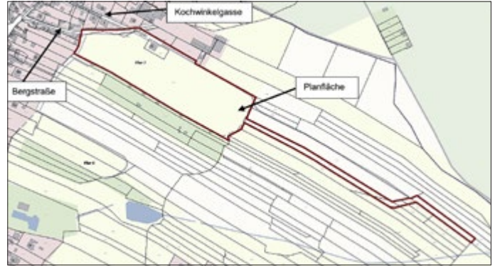
Geoproxy Thüringen (Zugriff 09.08.2022) Übersichtsplan - Geltungsbereich des Bebauungsplanes (unmaßstäbliche Darstellung)
